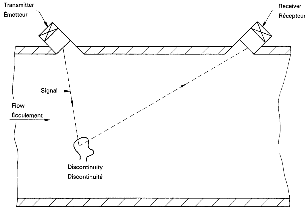
Figure 30 — Principle of operation of the Doppler ultrasonic meter Figure 30 — Principe de fonctionnement d'un débitmètre à ultrasons à effet Doppler
