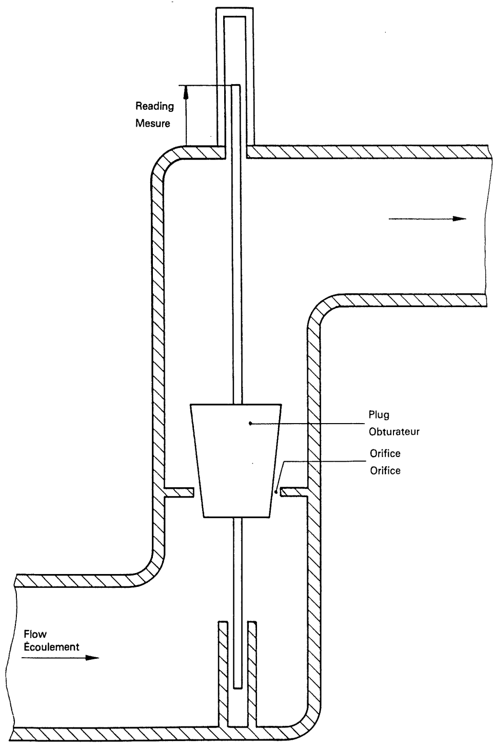
Figure 23 — Orifice-and-plug meter Figure 23 — Débitmètre à obturateur
