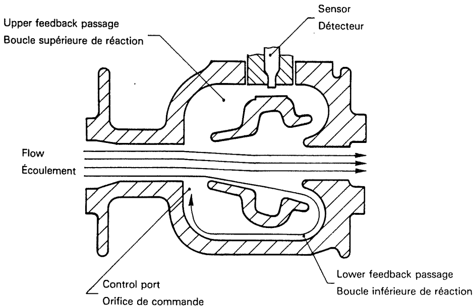
Figure 17 — Principle of operation of a fluidic flowmeter, shown with the flow in one of the two alternative modes Figure 17 — Principe de fonctionnement d'un débitmètre fluidique représenté avec le fluide s'écoulant dans l'un des deux modes possibles
