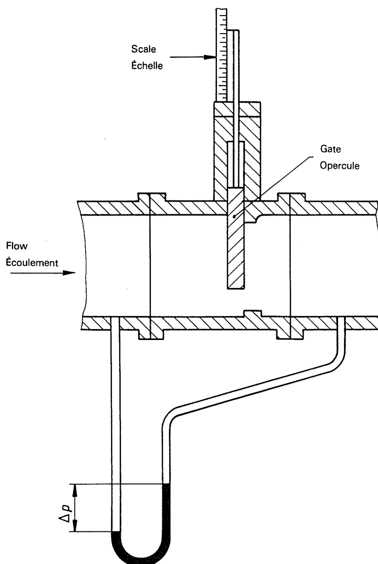
Figure 24 — Gate-type meter Figure 24 — Débitmètre à opercule
