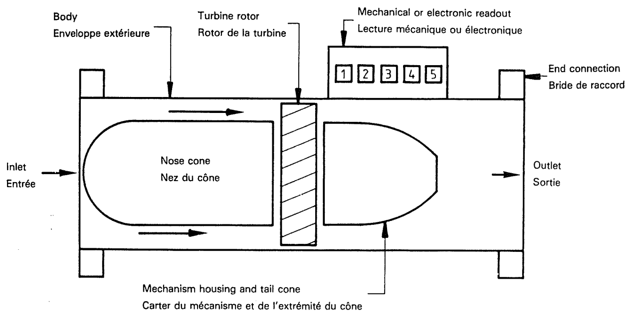
Figure 32 — Gas turbine meter Figure 32 — Compteur de gaz à turbine
