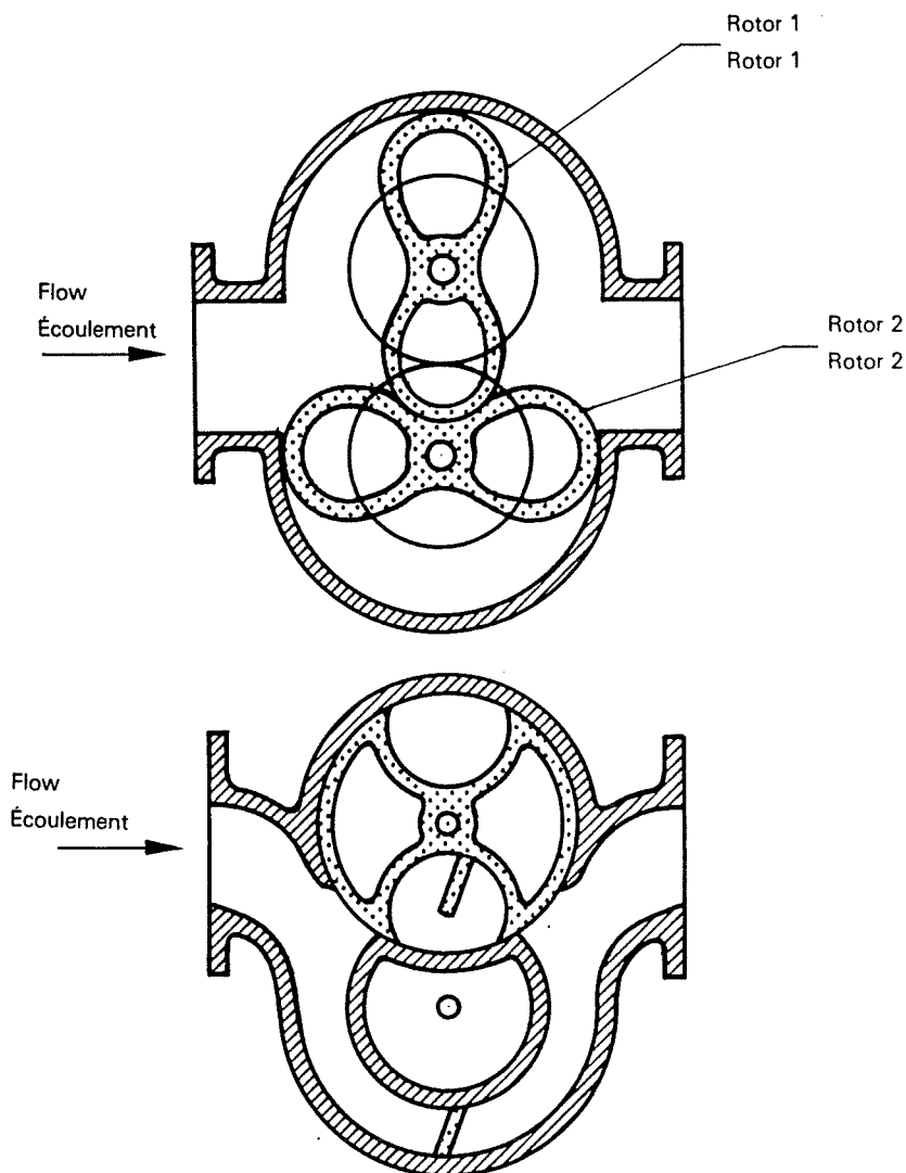
Figure 31 — Examples of rotary displacement meters Figure 31 — Exemples de compteurs volumétriques rotatifs
