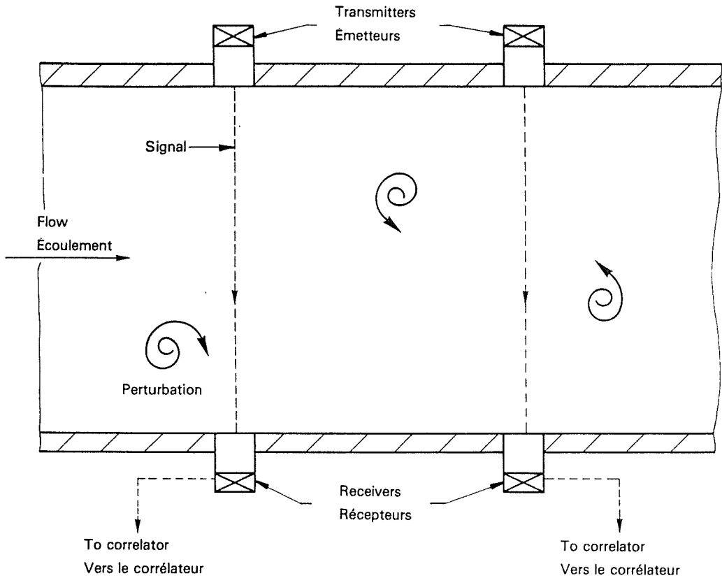
Figure 29 — Principle of operation of the cross-correlation ultrasonic meter Figure 29 — Principe de fonctionnement d'un débitmètre à ultrasons à intercorrélation
