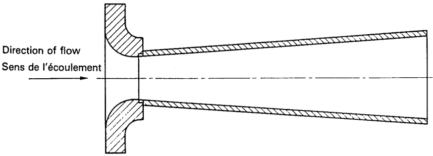
Figure 8 — Toroidal throat Venturi nozzle Figure 8 — Venturi-tuyère à col toroïdal
