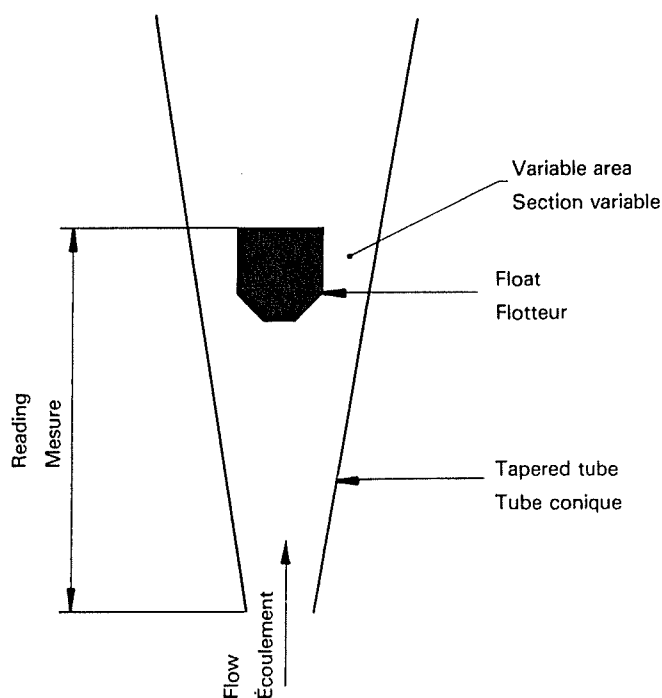
Figure 22 — Principle of operation of a cone-and-float meter Figure 22 — Principe du débitmètre conique à flotteur
