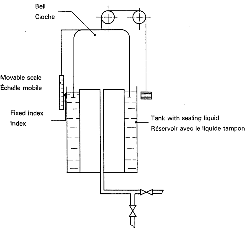
Figure 13 — Bell prover Figure 13 — Jaugeur à cloche (gazomètre)
