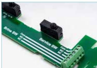
Micro-switches auxiliaires
