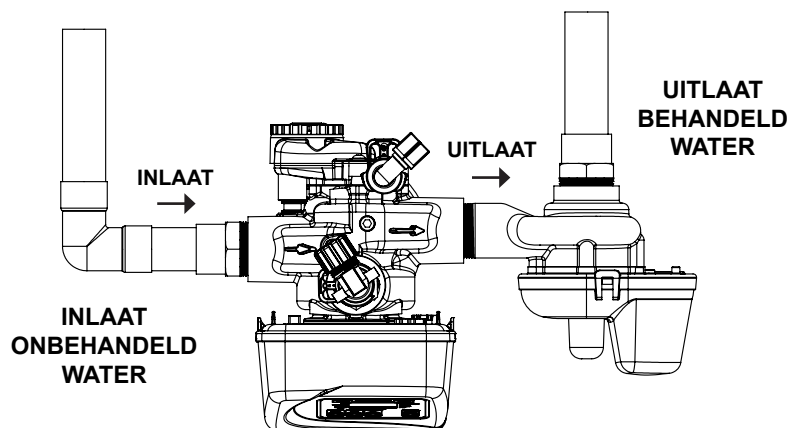
VOORBEELD VAN EEN NHWBP-CONFIGURATIE
